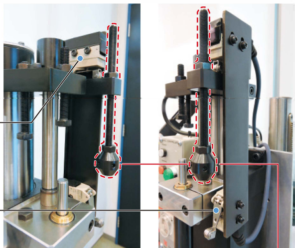
ドグ・ドグバー (LSキットの単品注文の時には付属されておりません) Dog and dog bar (It is not included when you buy LS KIT only).
